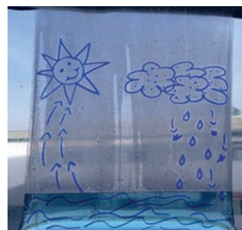
Ciclo hidrológico
